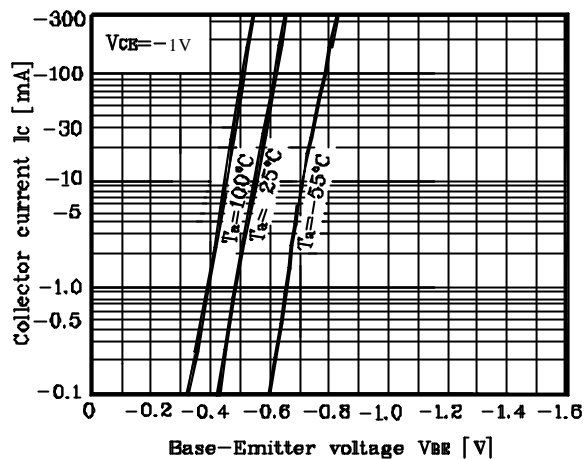
Fig. 2 I_C - V_{BE}
